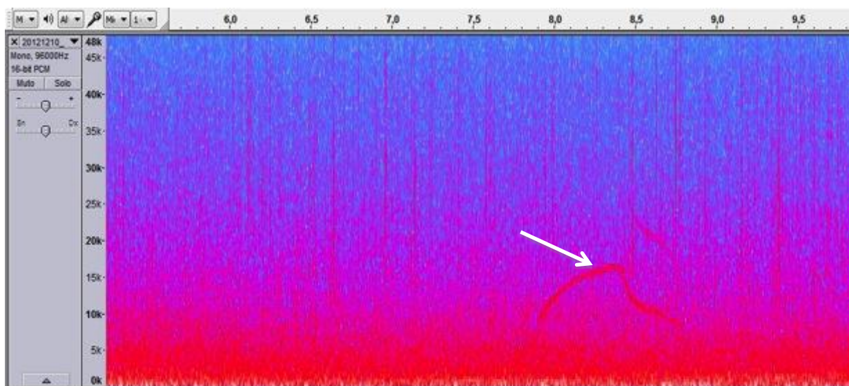
Figura 7. Whistle ('fischii') di delfini registrati il 10 dicembre alle ore 09:04 (indicati dalla freccia bianca) presso la stazione acustica 7. L'asse delle ordinate mostra la frequenza in kHz, mentre l'asse delle ascisse rappresenta il tempo in millisecondi.
